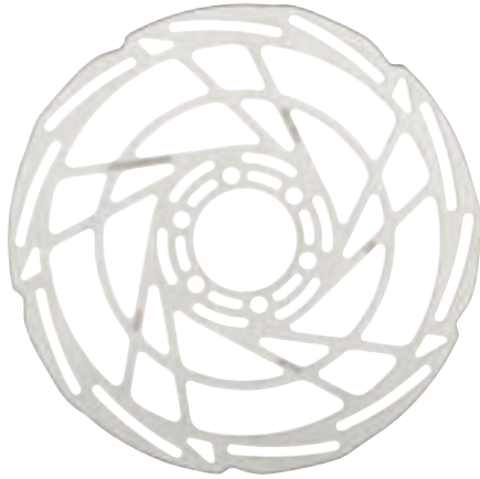
DCR043 6-Bolt Disc - 203mm - 192g
